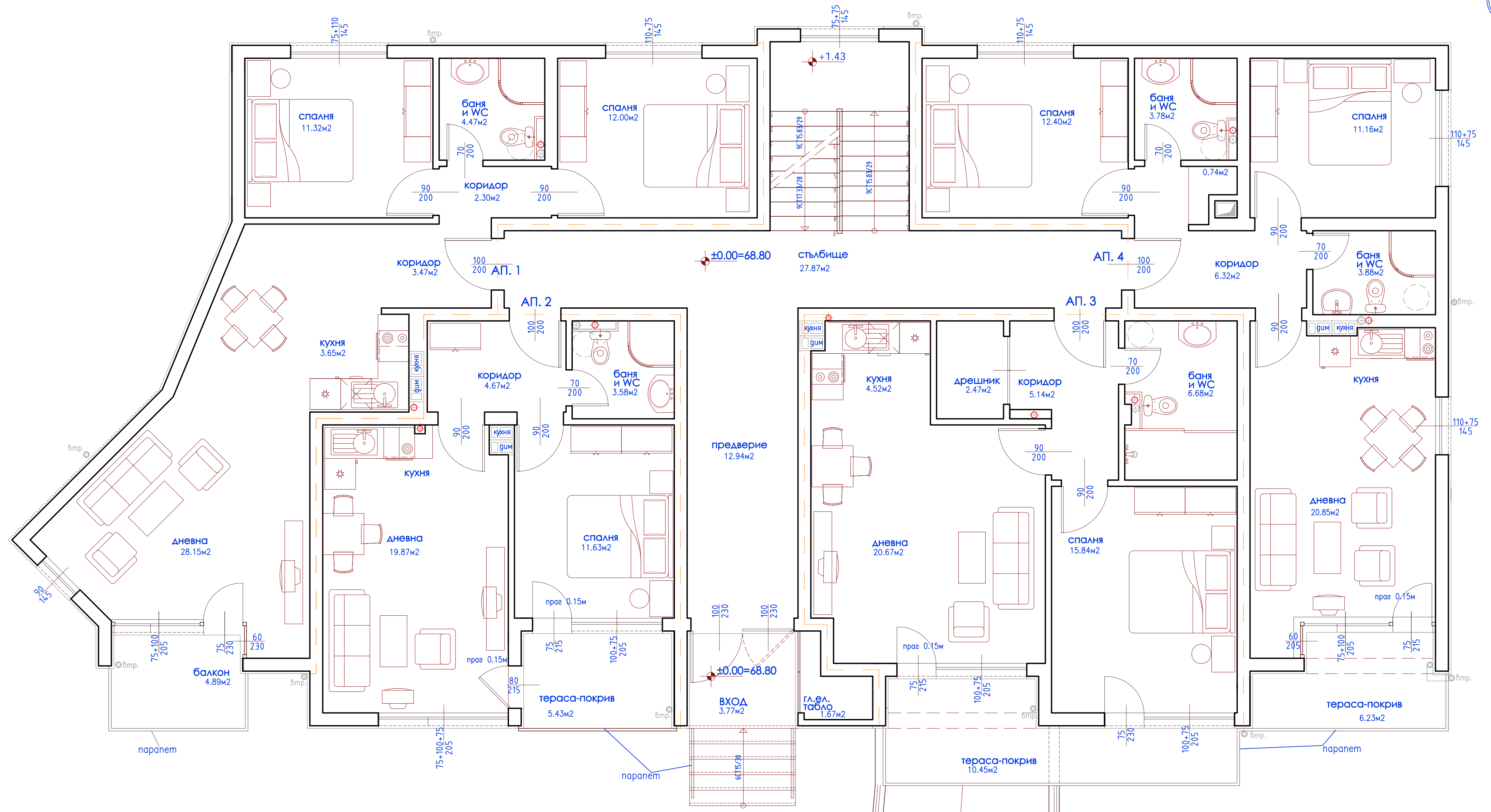
ПЪРВИ ЕТАЖ ПЛАН М 1:50
