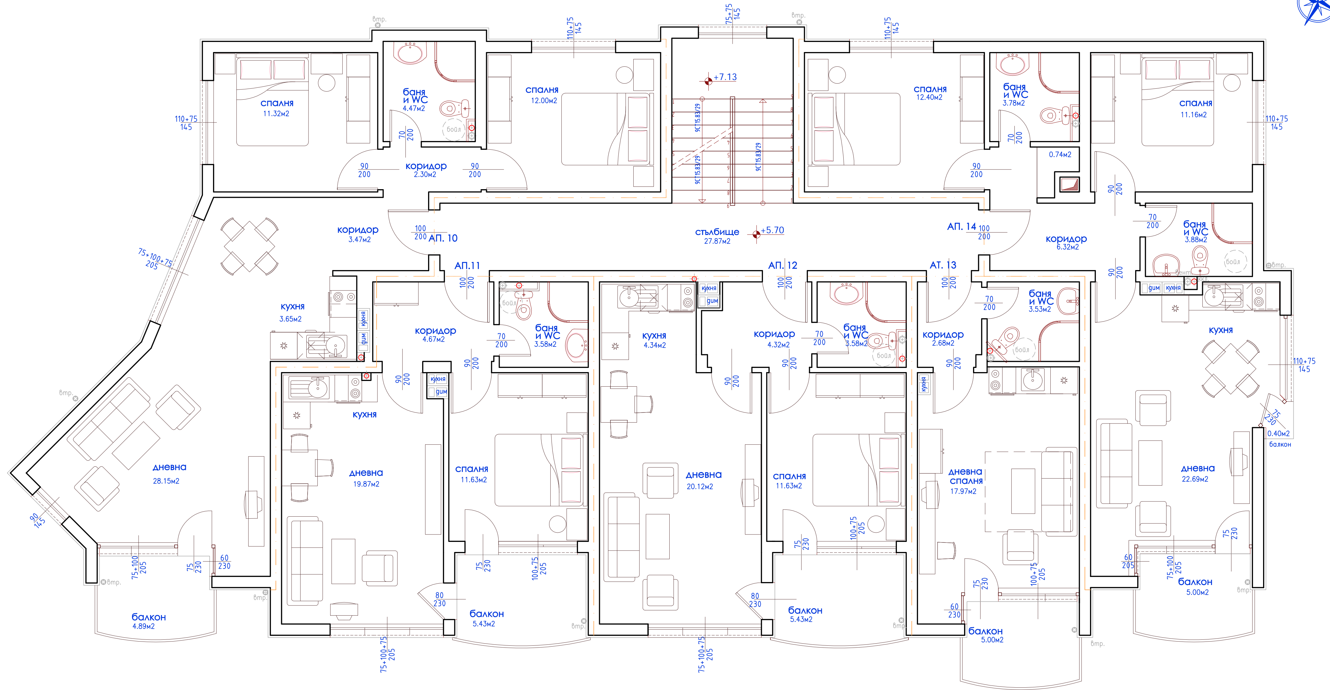
ТРЕТИ ЕТАЖ ПЛАН М 1:50
